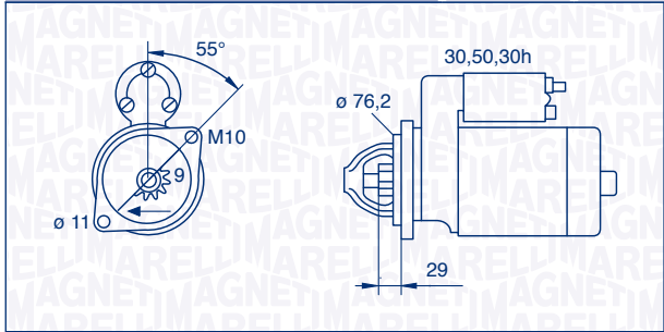
063521081960 – MSN2201 1,4 kW 12 V
