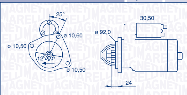
063280020010 – MSN8020 2,3 kW 12 V
