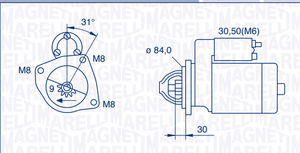
063521093070 – MSN2009 2,3 kW 12 V
