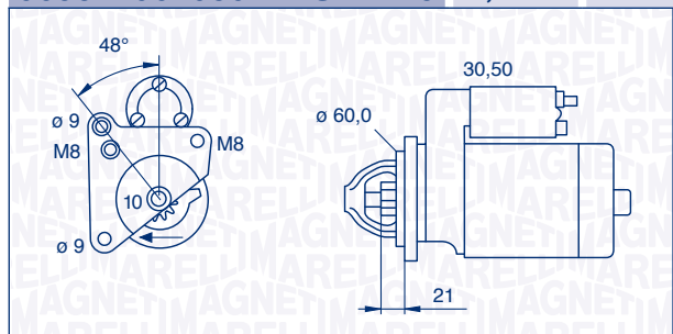
063521064050 – MSN2123 0,9 kW 12 V
