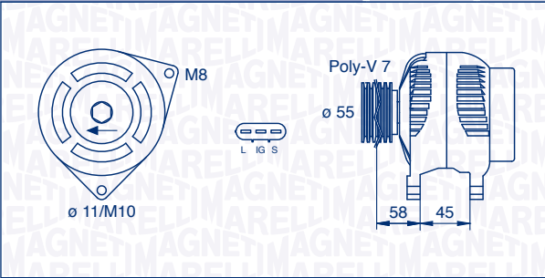
063377434010 – MAN7434 90 A 12 V
