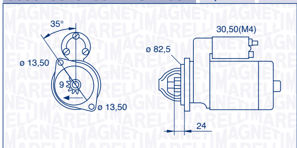
063523620760 – MSN2051 2,4 kW 12 V
