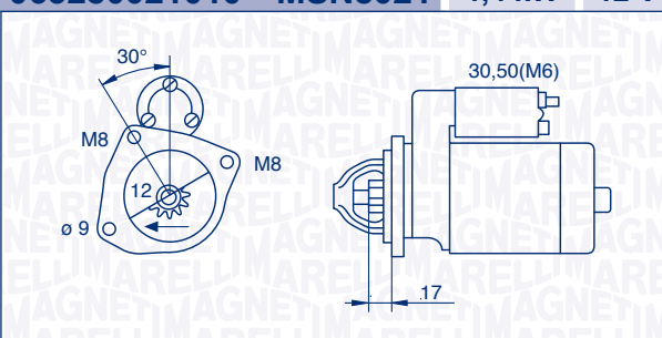
063280021010 – MSN8021 1,4 kW 12 V
