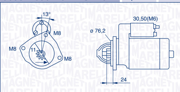
063521090110 – MSN2021 1,6 kW 12 V
