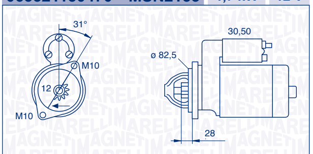
063521150470 – MSN2153 1,7 kW 12 V
