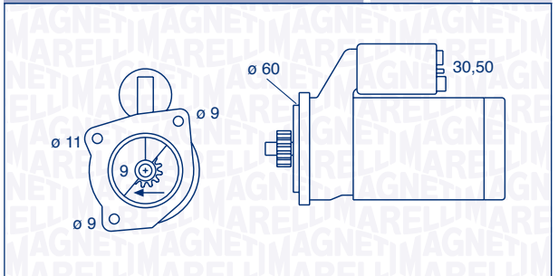
063523628010 – MSN3628 2,0 kW 12 V
