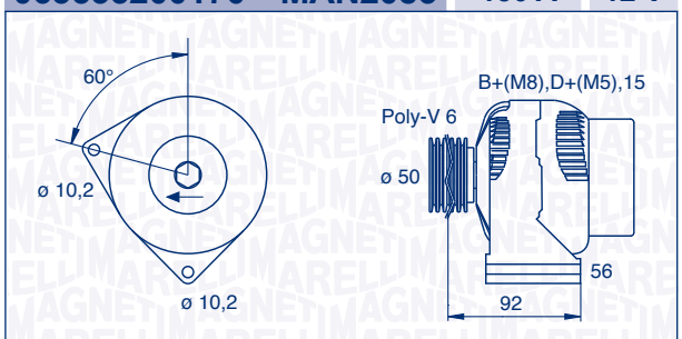
063535200170 – MAN2083 150 A 12 V
