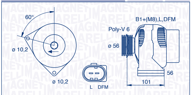
063535150460 – MAN2086 120 A 12 V
