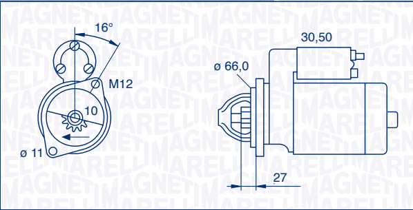
063521150820 – MSN2156 1,7 kW 12 V
