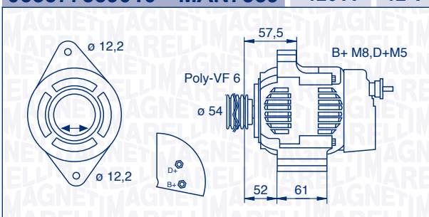
063377559010 – MAN7559 120 A 12 V
