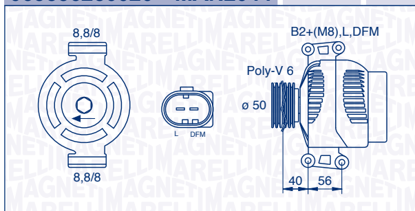
063536250020 – MAN2044 200 A 12 V
