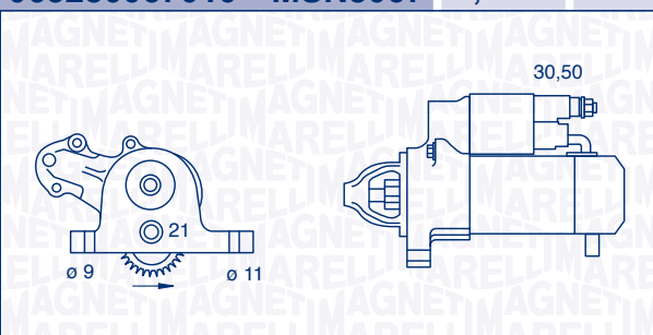
063280067010 – MSN8067 2,2 kW 12 V
