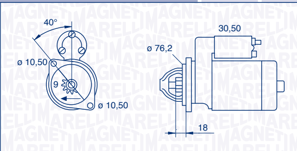
063521070620 – MSN2014 1,1 kW 12 V
