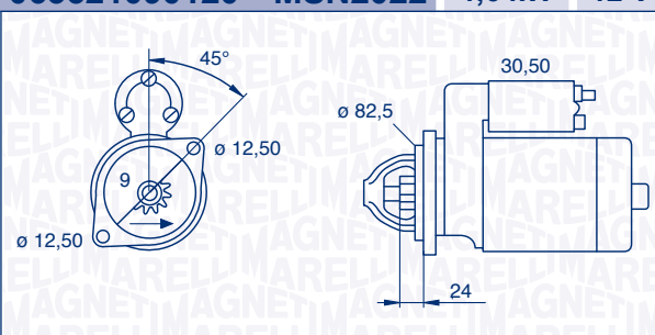
063521090120 – MSN2022 1,6 kW 12 V
