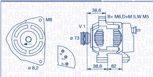
063377557010 – MAN7557 65 A 12 V
