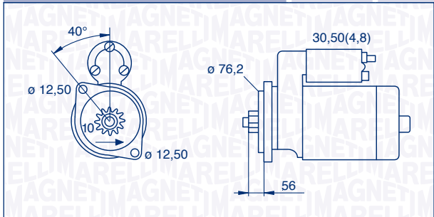
063521230180 – MSN2107 1,7 kW 12 V
