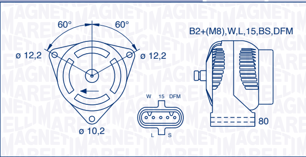
063536550090 – MAN2096 110 A 24 V
