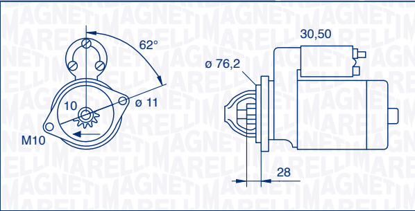
063521092580 – MSN2142 2,2 kW 12 V
