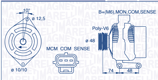
063377411010 – MAN7411 90 A 12 V
