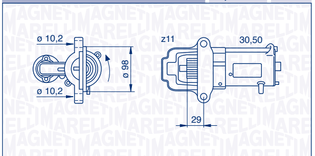
063280027010 – MSN8027 1,2 kW 12 V
