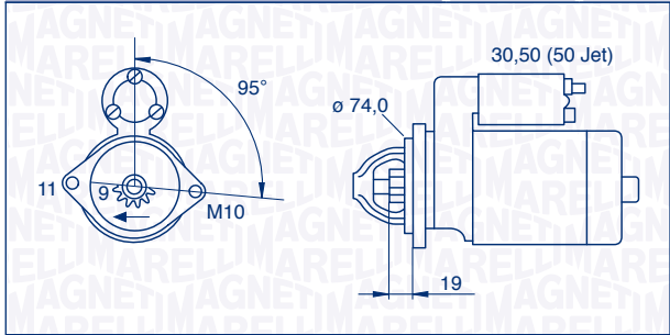
063280048010 – MSN8048 1,3 kW 12 V
