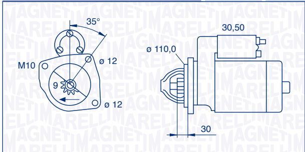
063521093440 – MSN2166 2,5 kW 12 V
