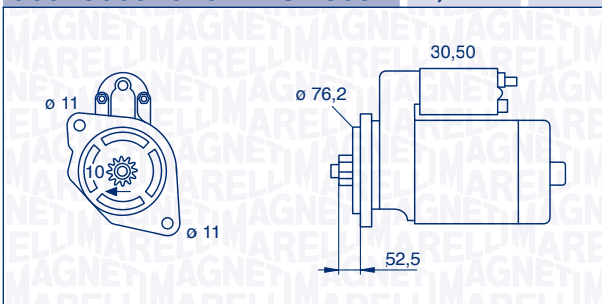
063280094010 – MSN8094 1,8 kW 12 V
