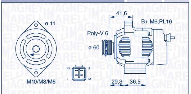
063377553010 – MAN7553 80 A 12 V
