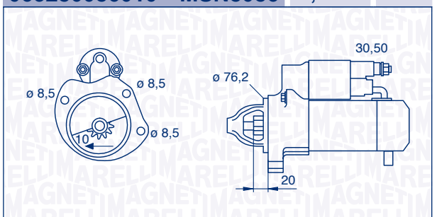
063280086010 – MSN8086 1,4 kW 12 V
