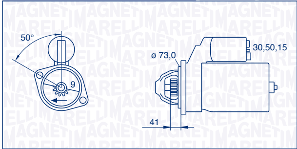
063226801010 – MSN139 1,4 kW 12 V
