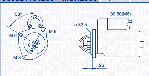
063521101250 – MSN2003 1,7 kW 12 V
