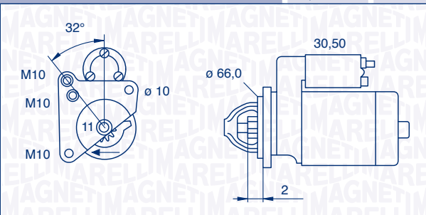
063521081860 – MSN2135 1,4 kW 12 V
