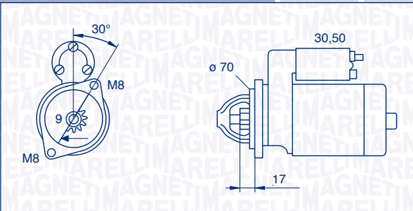
063191007010 – MSN800 0,8 kW 12 V
